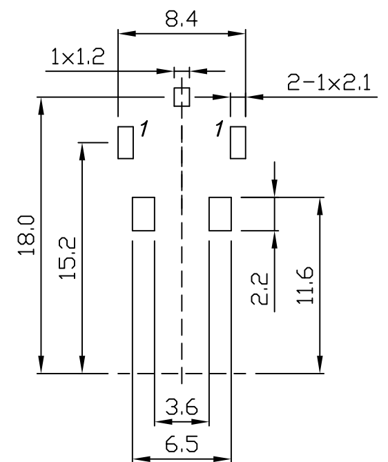
P.C.B LAYOUT(±0.1) (BOTTOM VIEW)
