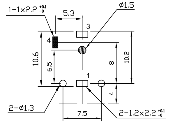
P.C.B LAYOUT(±0.1) (BOTTOM VIEW)
