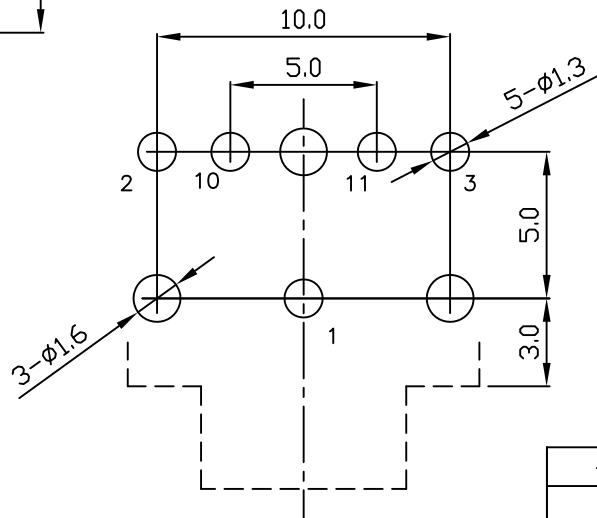
P.C.B LAYOUT(±0.1) (BOTTOM VIEW)
